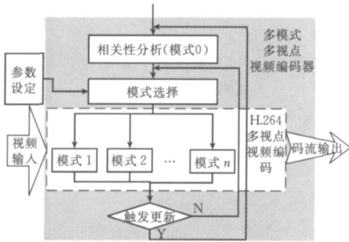
图 2 多模式多视点编码算法结构
