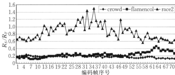
图 6 3 个多视点测试序列的相关性分析
