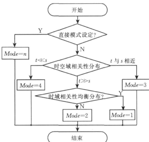
图 4 模式选择流程图
